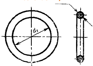
Кольца уплотнительные сечением 1,4 мм
